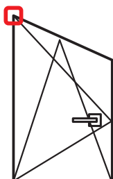
Anta singola apertura anta/ribalta a trapezio
