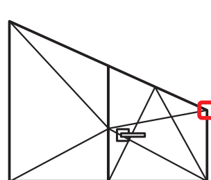
Anta primaria apertura anta/ribalta nei sistemi a trapezio a 2 ante
