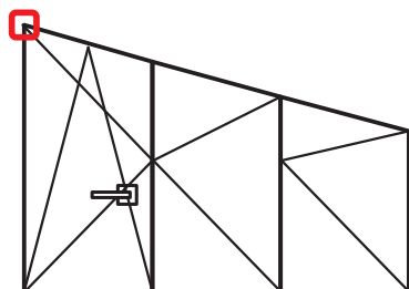
Anta primaria apertura anta/ribalta nei sistemi a trapezio a 3 ante
